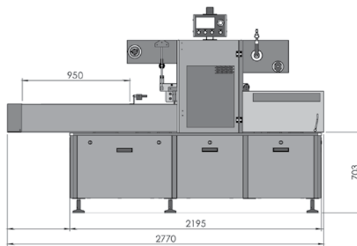
2 posizioni vaschetta 2 tray positions 2 Schalen Positionen
