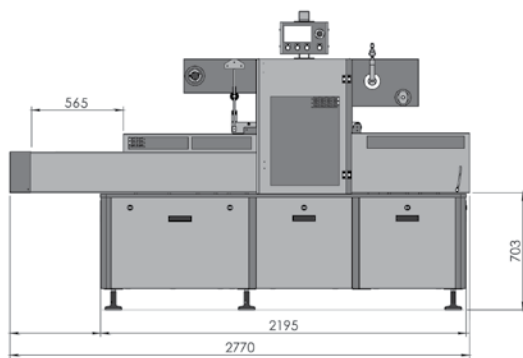
1 posizione vaschetta 1 tray position 1 Schalen Position
